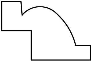
W-3020 1'' \times 1-1/2'' 1/2'' \times 1/2'' Rabbet
