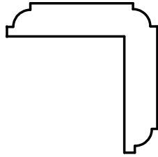
WM202 1-1/8" x 1-1/8"
