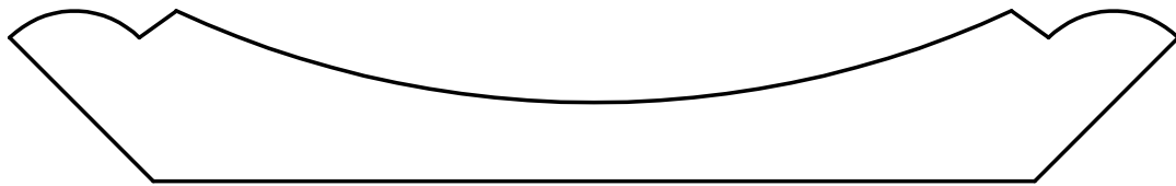
W-1598 13/16" x 5-9/16"
