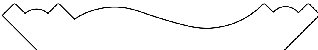
W-1469 13/16" x 5-9/16"
