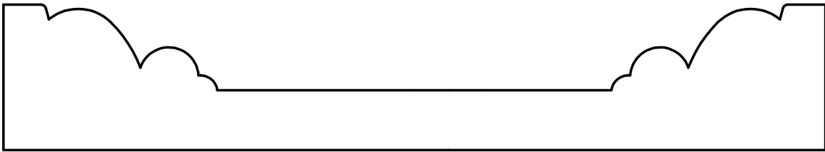
W-1169 1-1/16" x 6"
