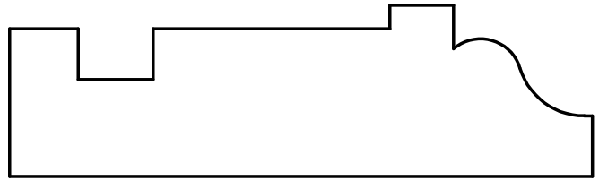
W-2076 1" x 3-3/8"
