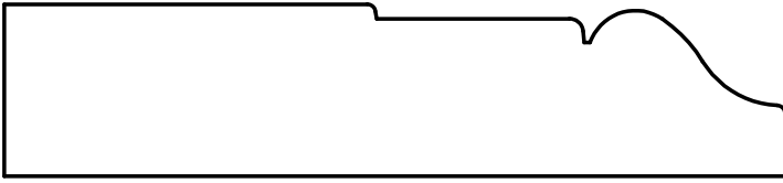
W-861 13/16" x 3-11/16"
